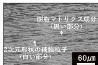
図1 試作試験体の断面観察像
