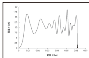
荷重－変位特性
