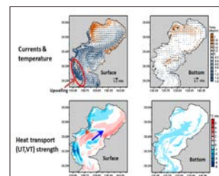
東京湾 超高解像度シミュレーション
